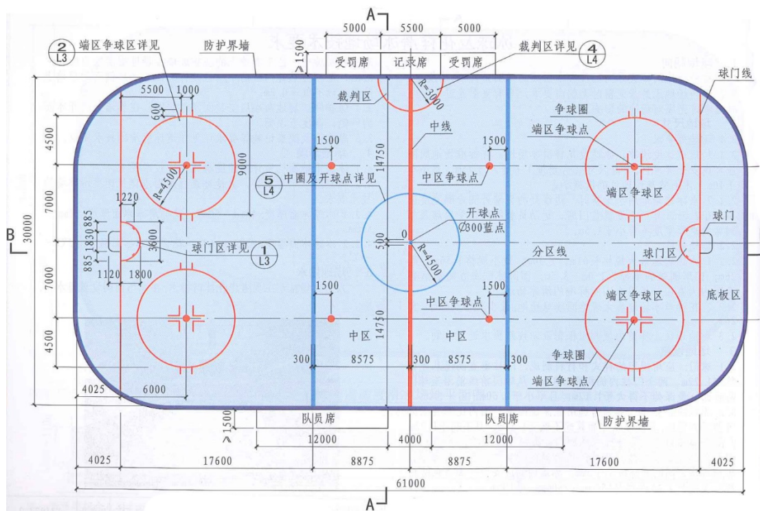
冰球场地平面图
