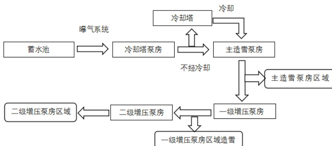
图5 造雪工艺系统供水流程图，需根据项目情况做针对性的设计
