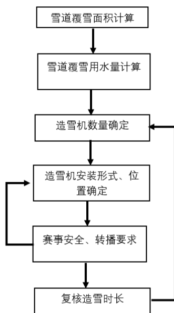
图 3 造雪设备的选型布置设计流程图
