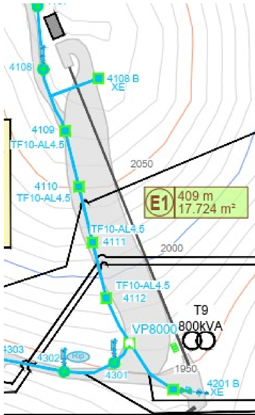
图 4 雪道及造雪机布置示意图
