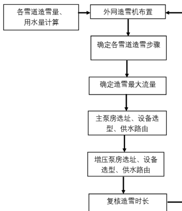
图6 造雪泵房设计流程图
