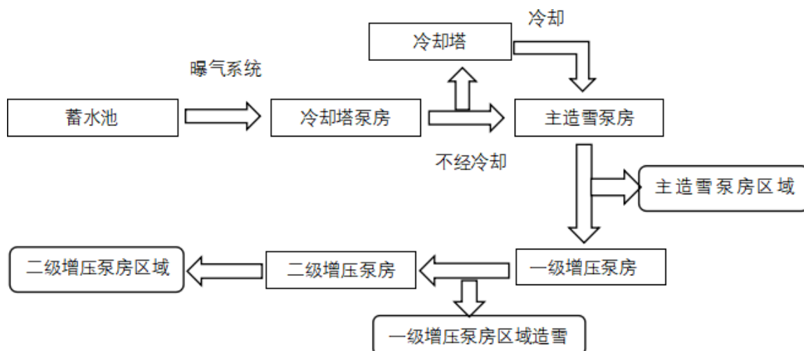
图5 造雪工艺系统供水流程图，需根据项目情况做针对性的设计
